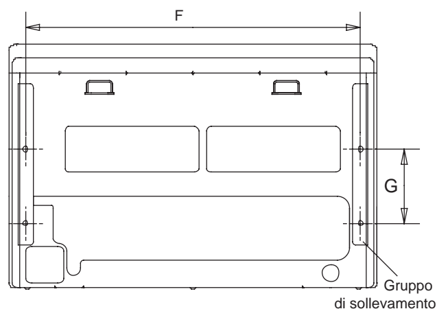
Dimensioni dei vari Modelli (unità: mm)
